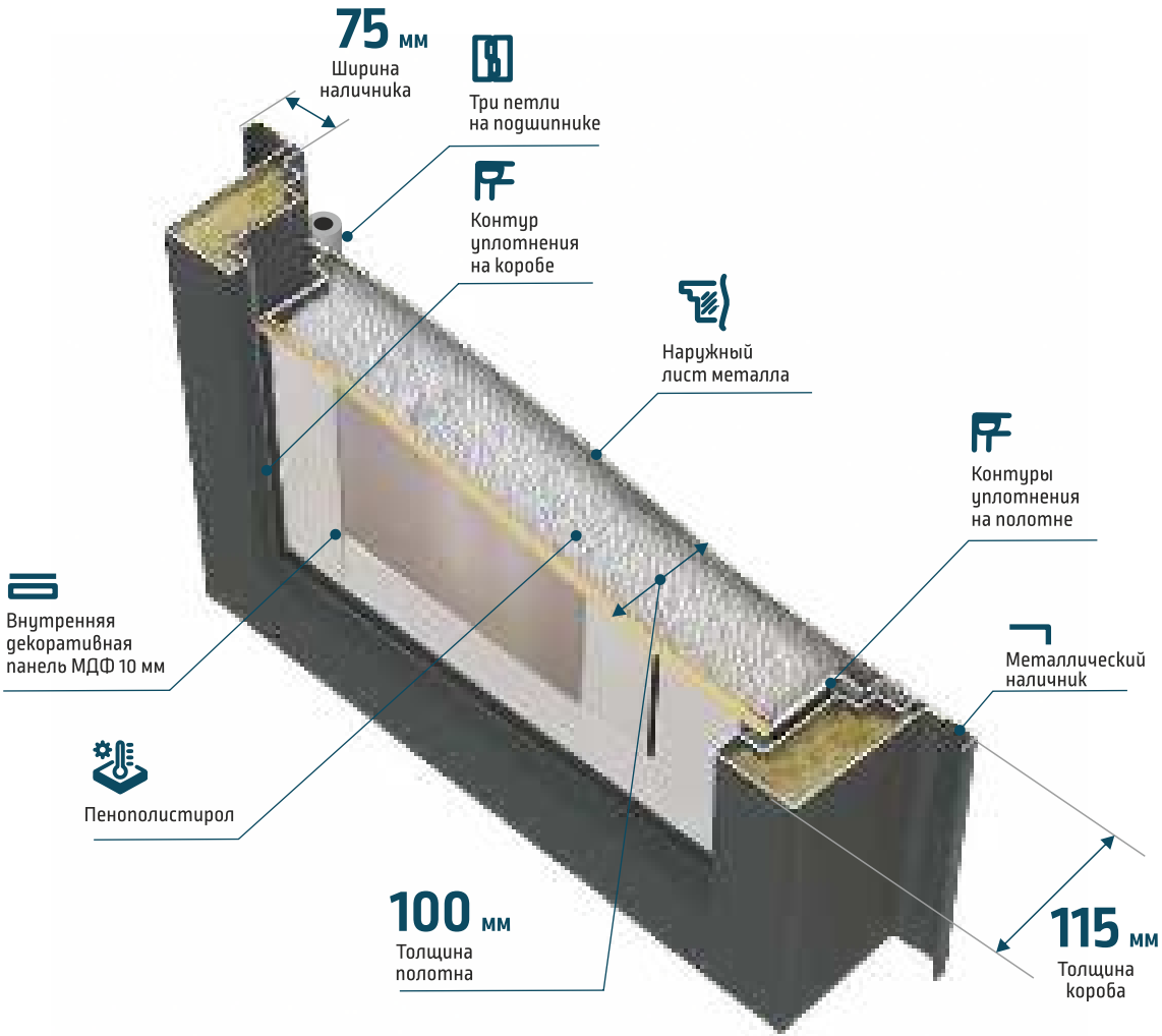
115 мм Короб закрытый 100 мм Толщина полотна 75 мм Ширина наличника
