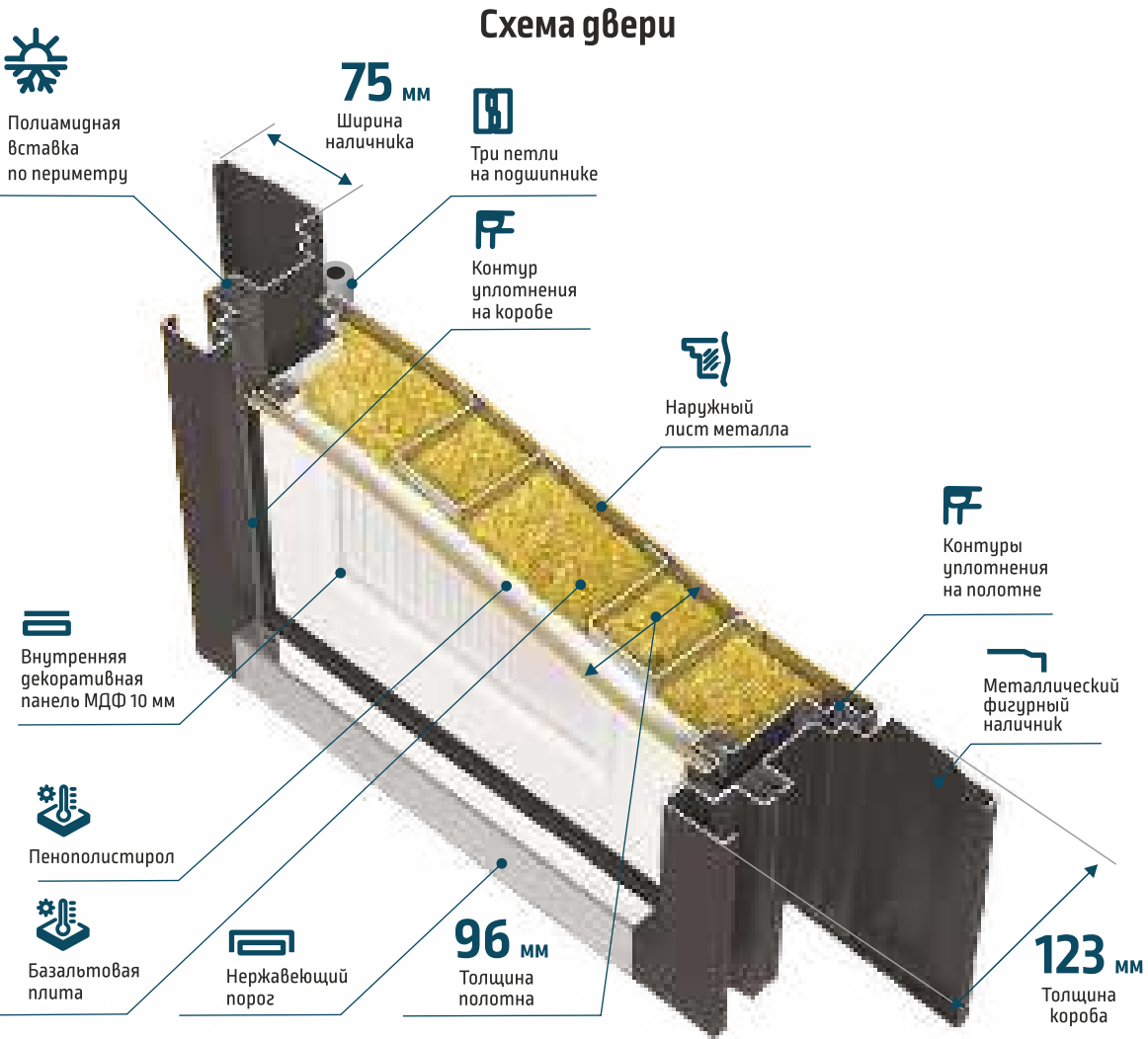
123 мм 96 мм 75 мм Короб открытый Толщина полотна Ширина наличника
